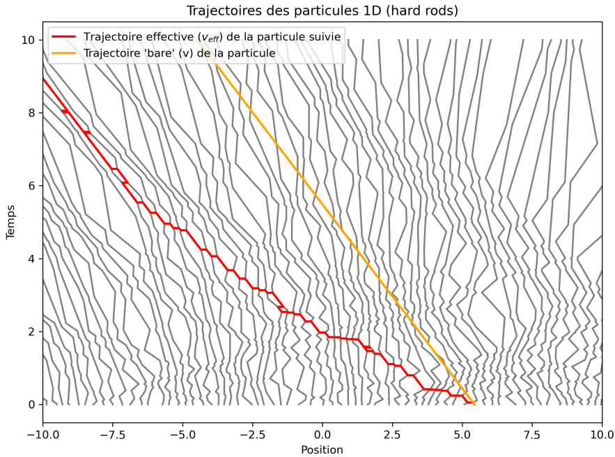
FIGURE 3.1 – Trajectoires des particules d'un gaz de hard rods en 1D. Les lignes noires représentent les particules individuelles, la ligne rouge correspond à la trajectoire effective (vitesse GHD) de la particule suivie, et la ligne orange indique la trajectoire de la particule si elle conservait sa vitesse initiale (bare velocity).
